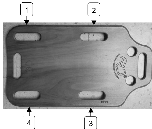
Detalle puntos de apoyo ensayo carga estática
